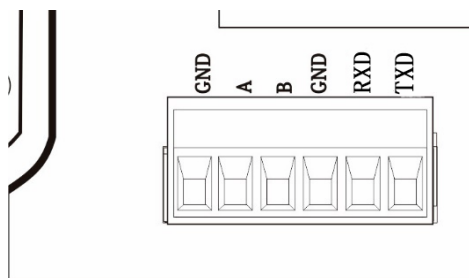
仪表与计算机连接图（ RS-232 方式）
