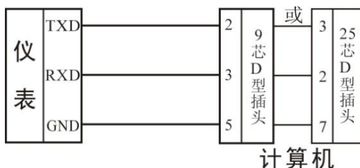
仪表与计算机连接图（ RS-232 方式）
